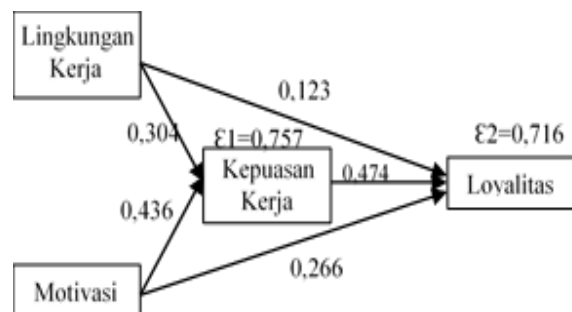
Gambar 2. Hasil olah Diagram Jalur Model Persamaan I dan II
